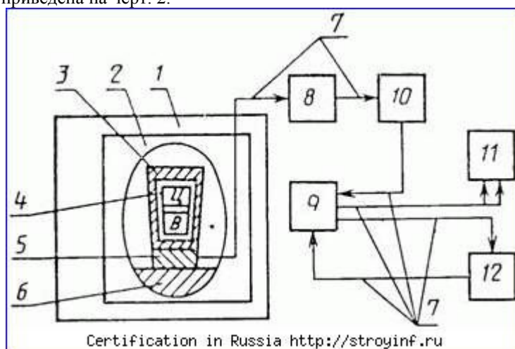
1-термостат; 2-калориметрический блок; 3-камера; 4-ячейка; 5-тепломер; 6-теплоотвод; 7-соединительные кабель; 8-коммутатор; 9-калибратор; 10-предварительный усилитель; 11-самописец; 12-интегратор
